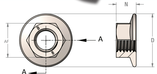
Flange Nut
